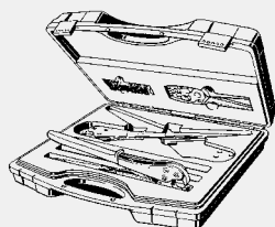
Pexfit Pro-Set de scule componente Clește de presat manual pentru diametrul de 16 mm, clește de presat manual pentru diametrul de 20 mm, dispozitiv de tăiat țevi d14-25, calibrator pentru diametrele 14-25, cutie model 4780.4
