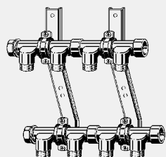
Distribuitoar - bronz - Rp-/R3/4 componente Suportii din oțel galvanizat, insertii izolatoare, ieșiri filetate pentru racordarea cu fittinguri Viega model 2005
