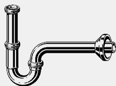
Sifon din țevi sifon Plus - alamă componente Țeavă prelungitoare 120 mm, cot de scurgere 220 mm controlat în privința calității conform normei EN 274 model 5611.5
