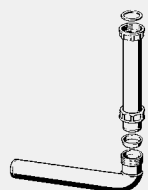
Cot de scurgere la 90° - plastic componente Țeavă de scurgere model 5632.2
